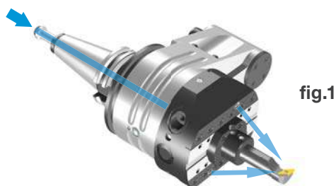
Adduzione liquido refrigerante fig.1
