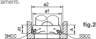
fig. 2 con un seggio SSCC ed un seggio SMCC disallineato e su un diverso diametro per operazioni di sgrossatura con alte profondità di passata.
