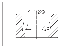
Due taglienti sullo stesso diametro
