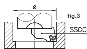
fig.3 con un solo seggio per operazioni di sgrossatura leggera o semifinitura.
